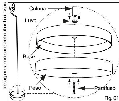
1º - Rosqueie a coluna na base.
