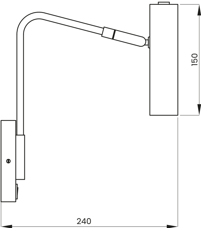
VISTA LATERAL
