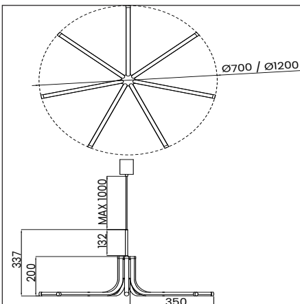
Desenho Técnico
