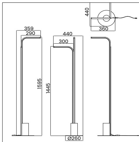
Desenho Técnico
